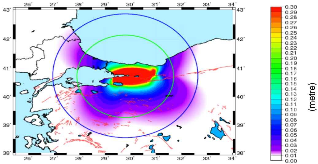
Şekil 5. İzmit Depreminin etki alanı. Daireler 160 ve 240 km'lik etki alanlarını göstermektedir. Yer değiştirme miktarı doğu, kuzey ve yükseklik bileşenlerinden en büyüğü alınarak metre cinsinden belirlenmiştir (Aktuğ vd., 2011).
