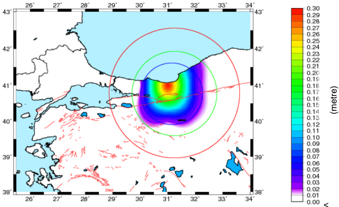
Şekil 6. Düzce Depreminin etki alanı. Yeşil ve mavi daireler sırasıyla 95, 130 ve 200 km'lik etki alanlarını göstermektedir. Yer değiştirme miktarı doğu, kuzey ve yükseklik bileşenlerinden en büyüğü alınarak belirlenmiştir (Aktuğ vd., 2011).
