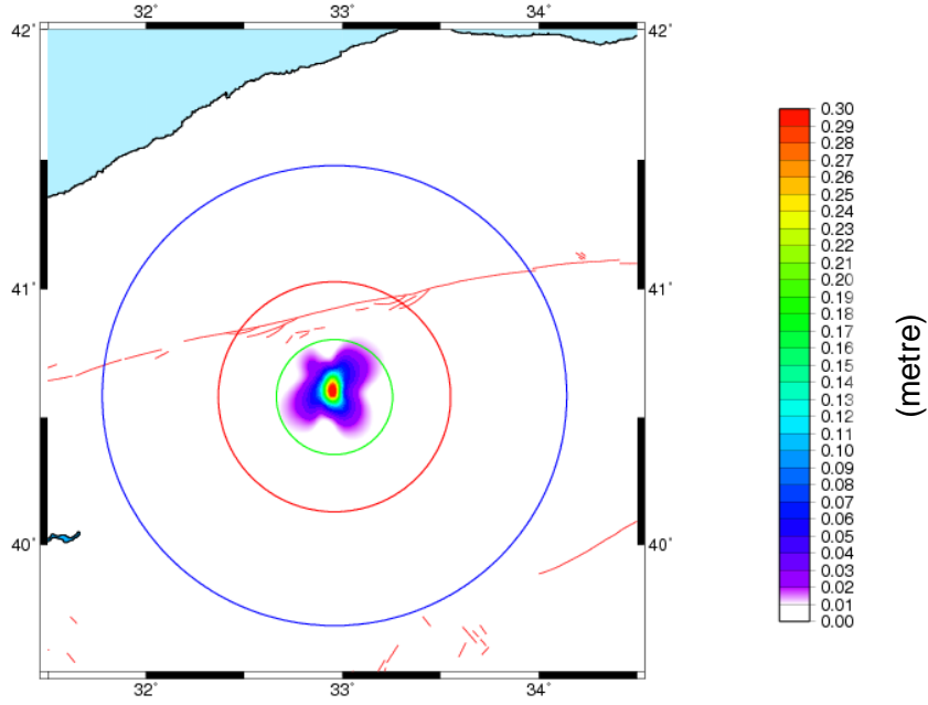
Şekil 7. 2000 Çerkeş Depreminin etki alanı. (Aktuğ, 2003)'de verilen eşitlikler ve (Taymaz vd., 2007)'de verilen inSAR çözümündeki fay geometrisi ve kayma değerleri ile hesaplanmıştır. Yer değiştirme miktarı doğu, kuzey ve yükseklik bileşenlerinden karelerinin toplamının karekökü şeklinde hesaplanmıştır. Mavi, kırmızı ve yeşil daireler sırasıyla 100, 50 ve 25 km yarıçaplı etki alanlarını göstermektedir (Aktuğ vd., 2011).
